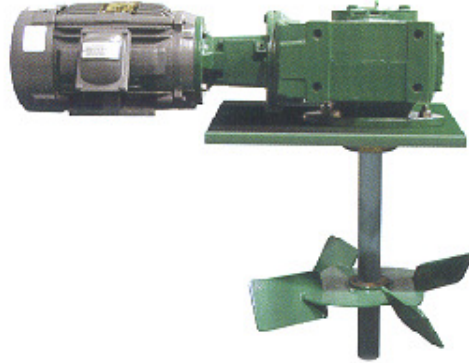
Agitador de lama horizontal
